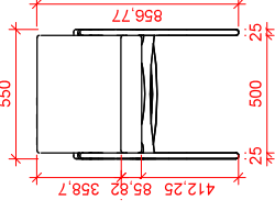
3 FRONTAL - ITEM 43 1 : 25
