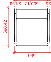
2 SUPERIOR - ITEM 43 1 : 25
